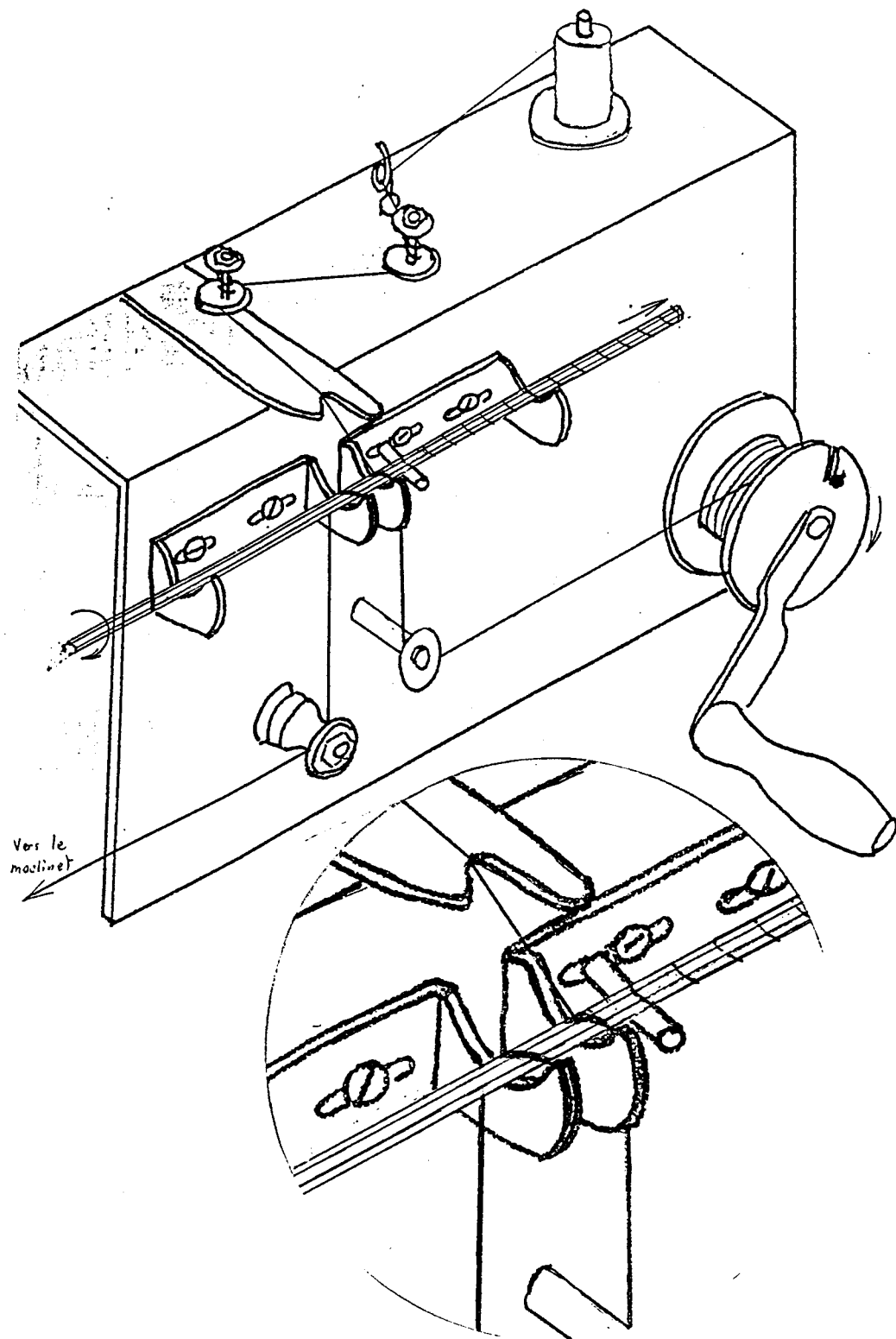
Croquis 3 Passage du cable en position "tourne à droite".
